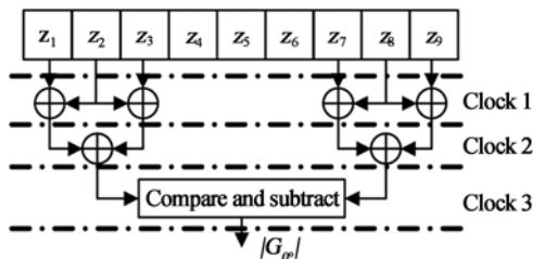
图 6 水平方向梯度计算结构图
