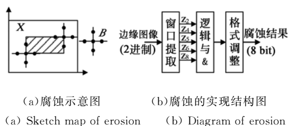
图 7 腐蚀运算实现过程
