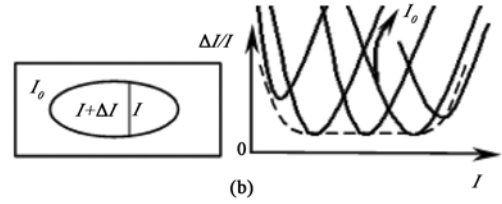
(b) 不同环境亮度下的 TVI 曲线
