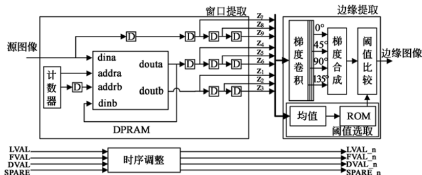
图 5 改进 Sobel 边缘检测实现结构图
