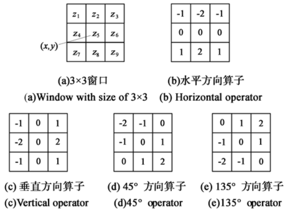
图 1 Sobel 算子
