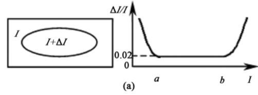
(a) 基本 TVI 比曲线
