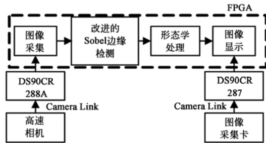
图 4 系统结构框图
